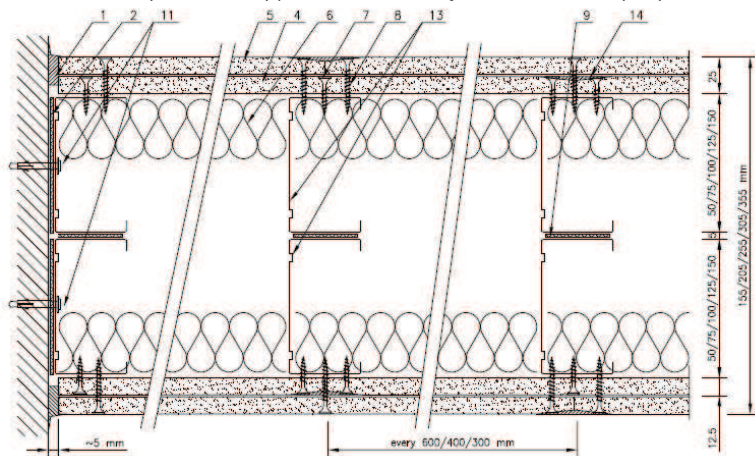
Rysunek Nr 2. Przekrój pionowy i poziomy antywłamaniowej nienośnej ściany działowej na szkielecie podwójnym (rzędy połączonych profili) z dwiema warstwami płyt.
