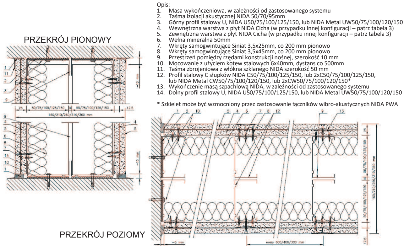
Rysunek Nr 3. Przekrój pionowy i poziomy antywłamaniowej nienośnej ściany działowej na szkielecie podwójnym (osobne rzędy profili) z dwiema warstwami płyt.
