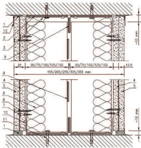
PRZEKRÓJ PIONOWY
