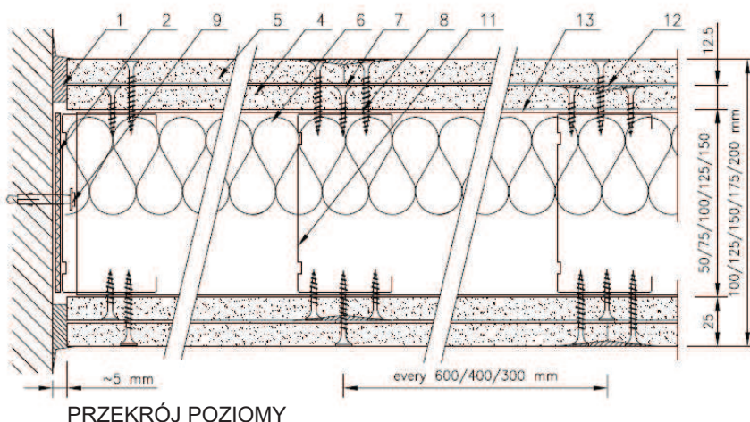
Rysunek nr 1. Przekrój pionowy i poziomy antywłamaniowej nienośnej ściany działowej na szkielecie pojedynczym z dwoma warstwami płyt.
