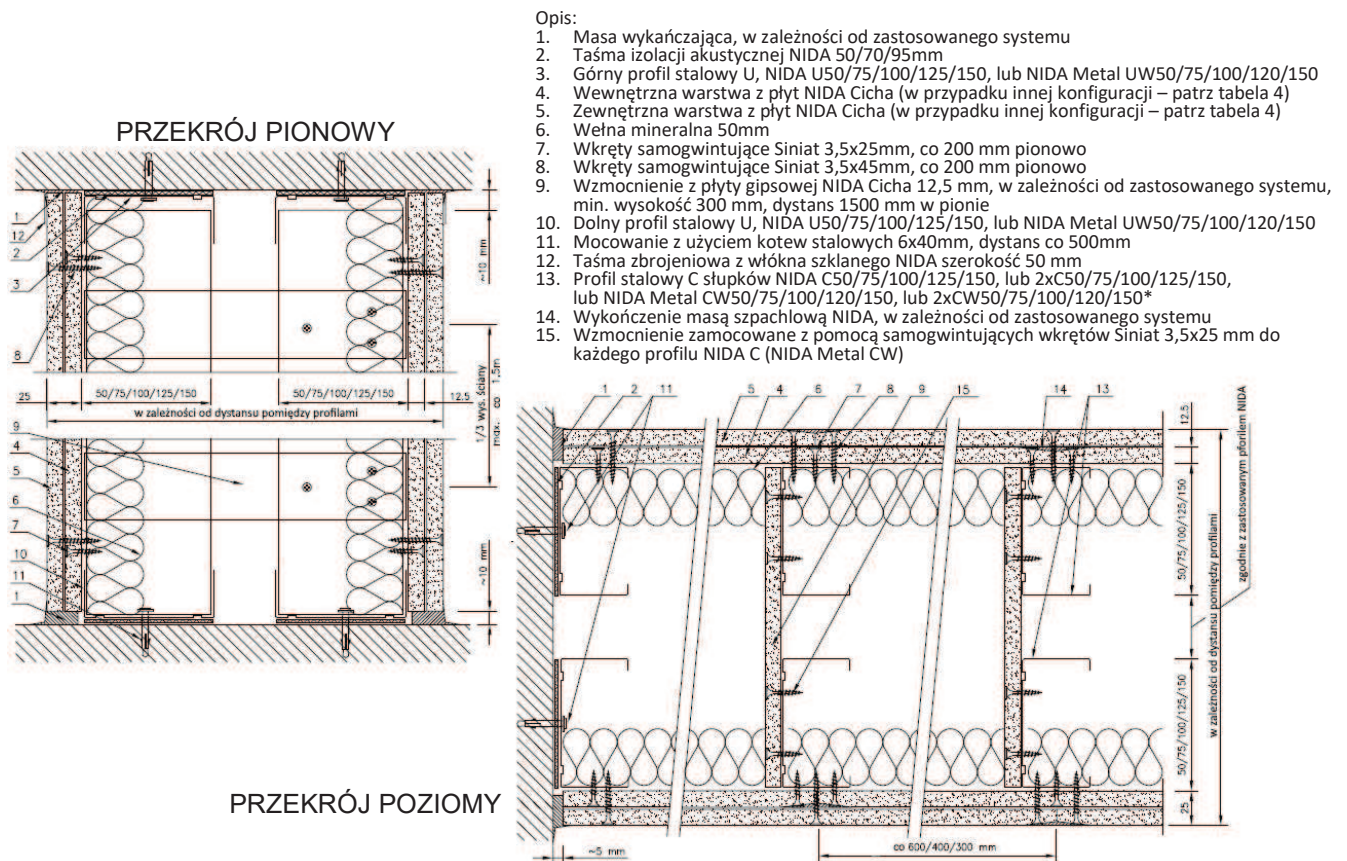
Rysunek Nr 4. Przekrój pionowy i poziomy antywłamaniowej nienośnej ściany działowej na podwójnym szkielecie i z dwiema warstwami płyt - do instalacji
