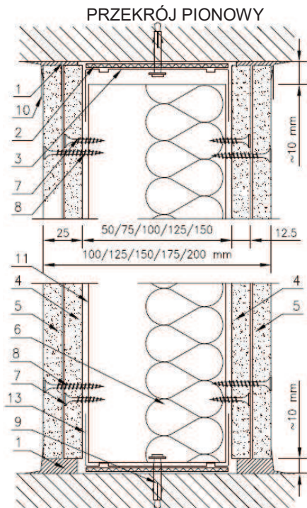
Rysunek nr 1. Przekrój pionowy i poziomy antywłamaniowej nienośnej ściany działowej na szkielecie pojedynczym z dwoma warstwami płyt.
